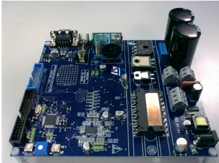
STEVAL-IHM034V2
