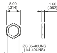
HEX NUT
