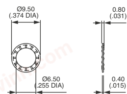
LOCKWASHER
