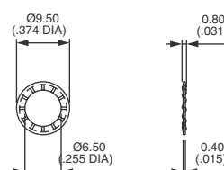
LOCKWASHER
