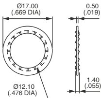
LOCKWASHER
